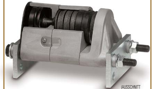
(AUSSCHNITT DES FS20 BREMSSATTELS ABGEBILDET)
