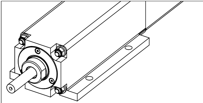
Abbildung 4.6: Die Konstruktion des GSWA33 Guided umfasst diese Baugruppe, die folgende Funktionen hat: Verdrehsicherung, Montagevorrichtung, seitliche Lastaufnahme.
