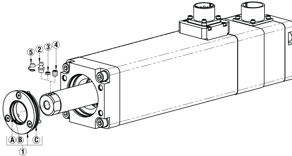
Abbildung 7.2: Explosionsdarstellung von GSWA33
