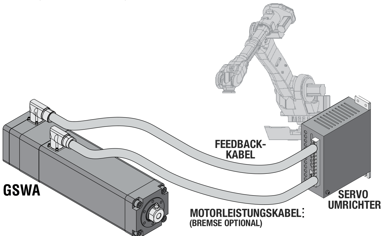
Abbildung 4.1: Typische Anschlüsse für ein einachsiges System mit einem ServoWeld™-Aktuator mit optionaler Bremse an einen RSW-Servosystemantrieb.
