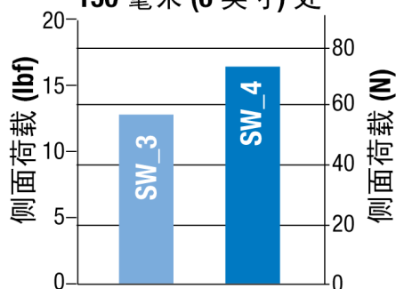
图 4.2：侧向载荷一定不要超过图中线条所表示的最大值
