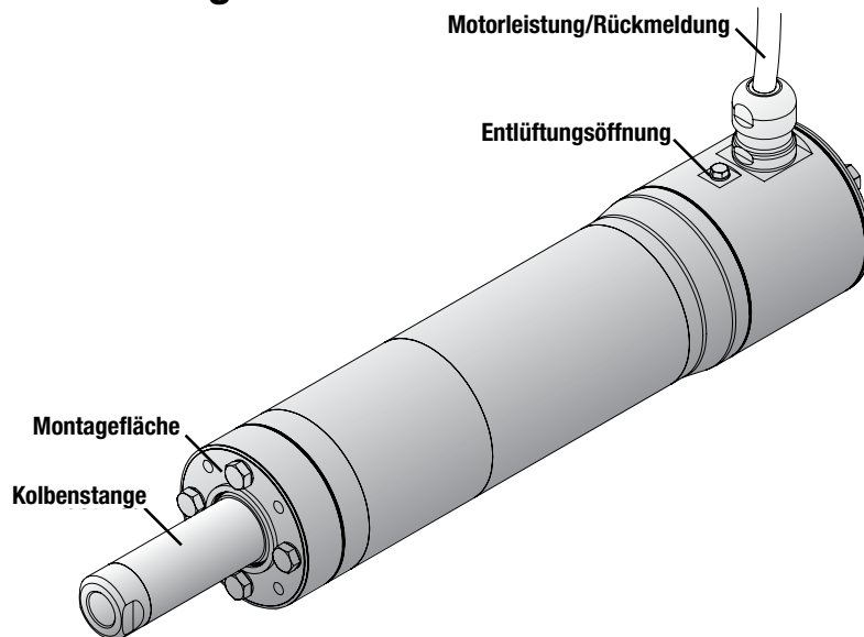
Abbildung 2-2 IMA-S Hauptkomponenten
