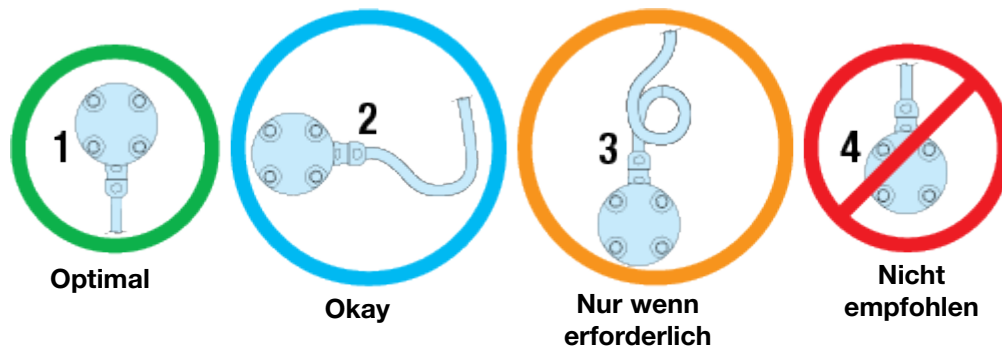
Abbildung 2-3: 1. Die bevorzugte Ausrichtung der Kabelverschraubung liegt unterhalb des Aktuators und erfordert keine Schleifen oder Biegungen. 2. Kabelverschraubungen an der Seite erfordern Biegungen oder Schleifen im Kabel. 3. Wenn sich die Kabelverschraubungen am oberen Ende des Aktuators befinden müssen, muss eine Schleife im Kabel hinzugefügt werden. 4. Kabelverschraubungen oben ohne Schleife werden nicht empfohlen.
