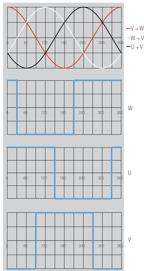
Abbildung 5-4: Hall-Ausrichtung
