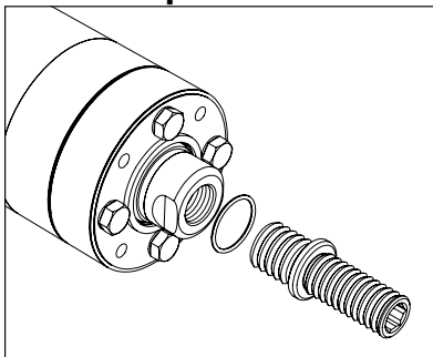
Abbildung 3-3 MET: Stangenkopf mit Außengewinde
