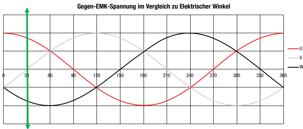
Abbildung 5-2: Gegen-EMK-Spannung im Vergleich zu Elektrischer Winkel
