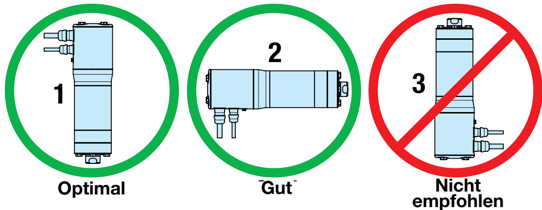
Abbildung 2-4: 1. und 2. Die empfohlene Ausrichtung der IMA-S-Kolbenstange ist nach unten oder horizontal. 3. Wegen der erhöhten Gefahr von Verschmutzung und Eindringen darf der IMA-S-Aktuator niemals mit der Kolbenstange nach oben ausgerichtet werden.
