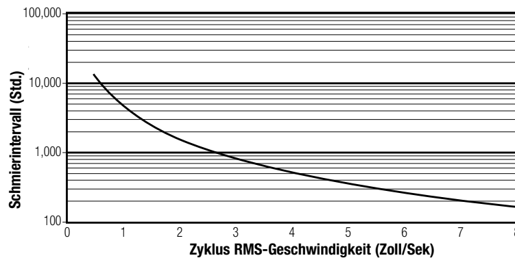
Abbildung 6-4: Diagramm der Rollengewindetriebe-Schmierintervalle
