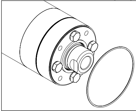
Abbildung 3-4 Standard-IMA-S-Halterung
