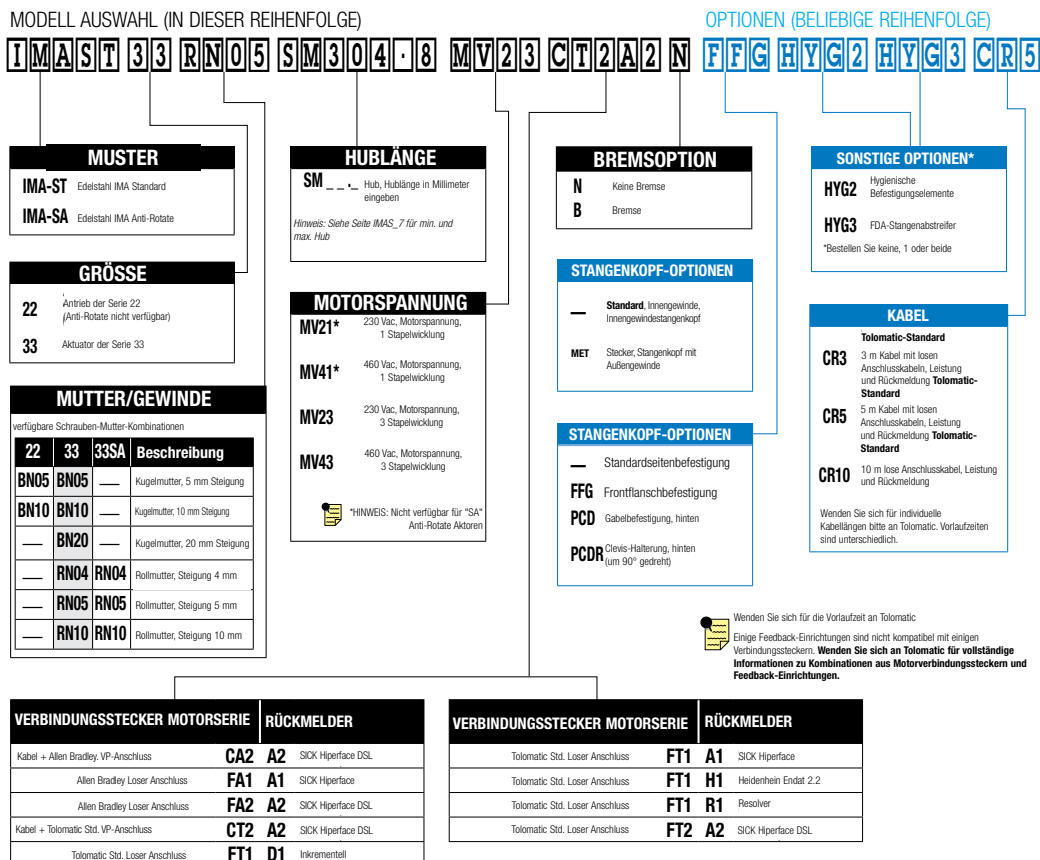
Abbildung 3-1 IMA-S Bestellcodes und Beschreibungen
