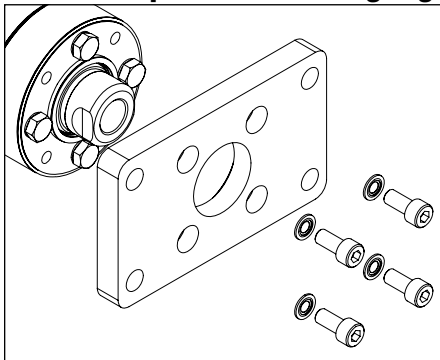
Abbildung 3-5 FFG: Frontflanscbefestigung
