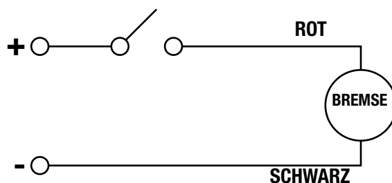
Abbildung 6-1: Schnellste Einrast-/Ausrastzeit, geringster Schutz
