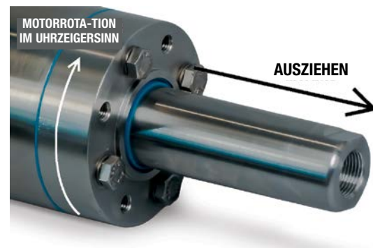
Abbildung 5-1: Kolbenstangenbewegung im Verhältnis zur Motorrotation
