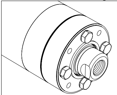
Abbildung 3-2 Standard-Innengewindestangenkopf
