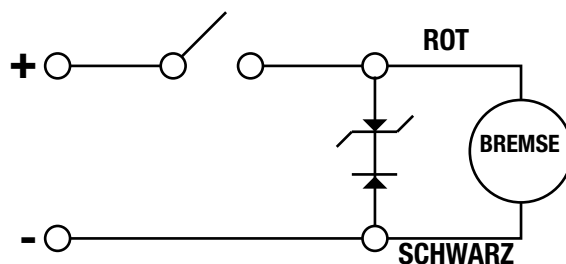
Abbildung 6-2: Erhöhte Aktivierungs-/Deaktivierungszeit, bester Schutz
