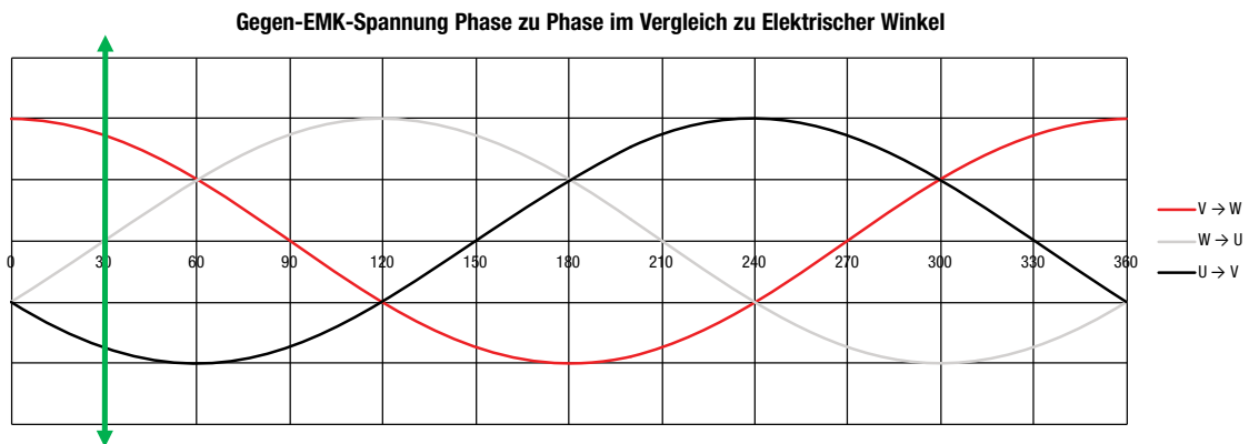
Abbildung 5-3: Gegen-EMK-Spannung Phase zu Phase im Vergleich zu Elektrischer Winkel
