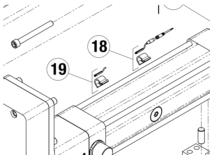
Abbildung 3-9 RSX Positionssensoren
