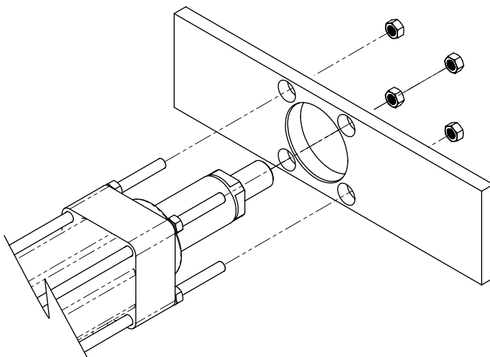
Abbildung 3-8 RSX verlängerte Zugstangen-Option
