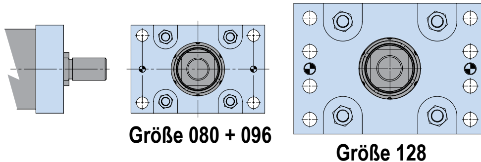
Abbildung 4-6 RSX Frontflansch-Option
