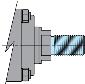
Abbildung 3-7 RSX Außengewinde-Option
