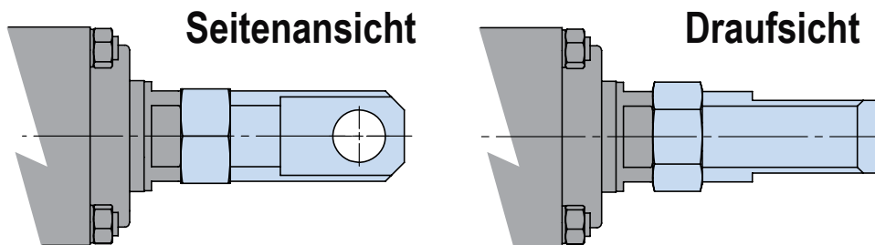
Abbildung 3-6 RSX-Gabelkopf-Option
