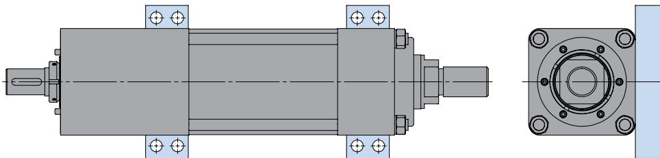
Abbildung 3-3 RSX Montageplatten-Option
