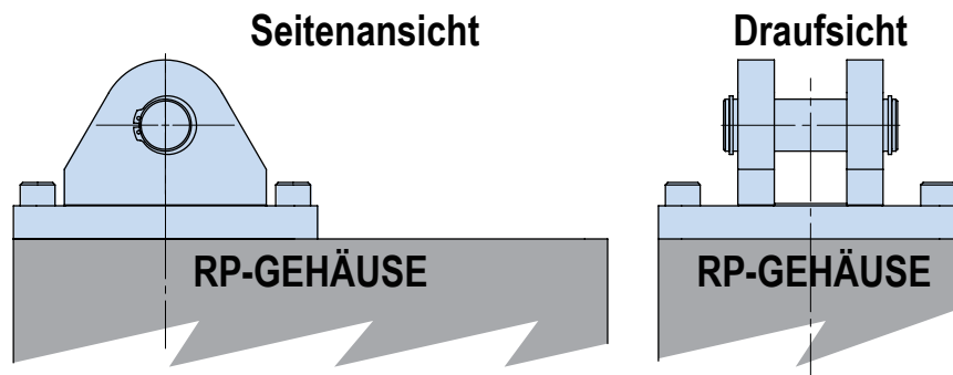
Abbildung 4-9 RSX Hinterteilhalterung auf Stellantrieb für parallel gegenläufige Motorhalterung
