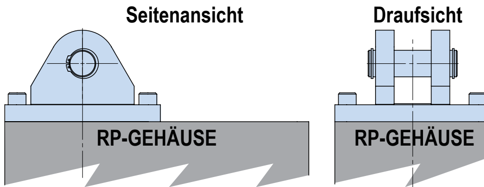
Abbildung 3-4 RSX Hinterteilhalterung auf Stellantrieb RP- Motorhalterung
