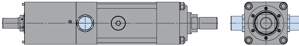
Abbildung 3-5 RSX Zapfenhalterungsoption
