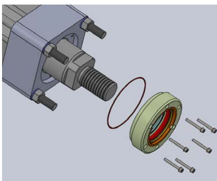
Abbildung 6-1 RSX-Dichtungspatrone Explosionsansicht
