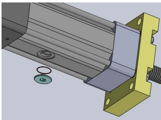
Abbildung 6-2 Explosionsansicht RSX-Schmierzugriffsabdeckung
