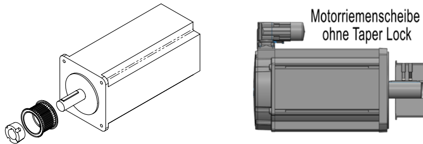
Abbildung 4-3 RSX RP Motor und Riemenscheibe
