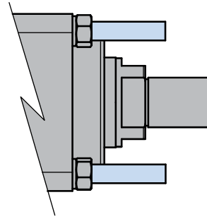
Abbildung 4-10 RSX verlängerte Zugstangenhalterungs-Option
