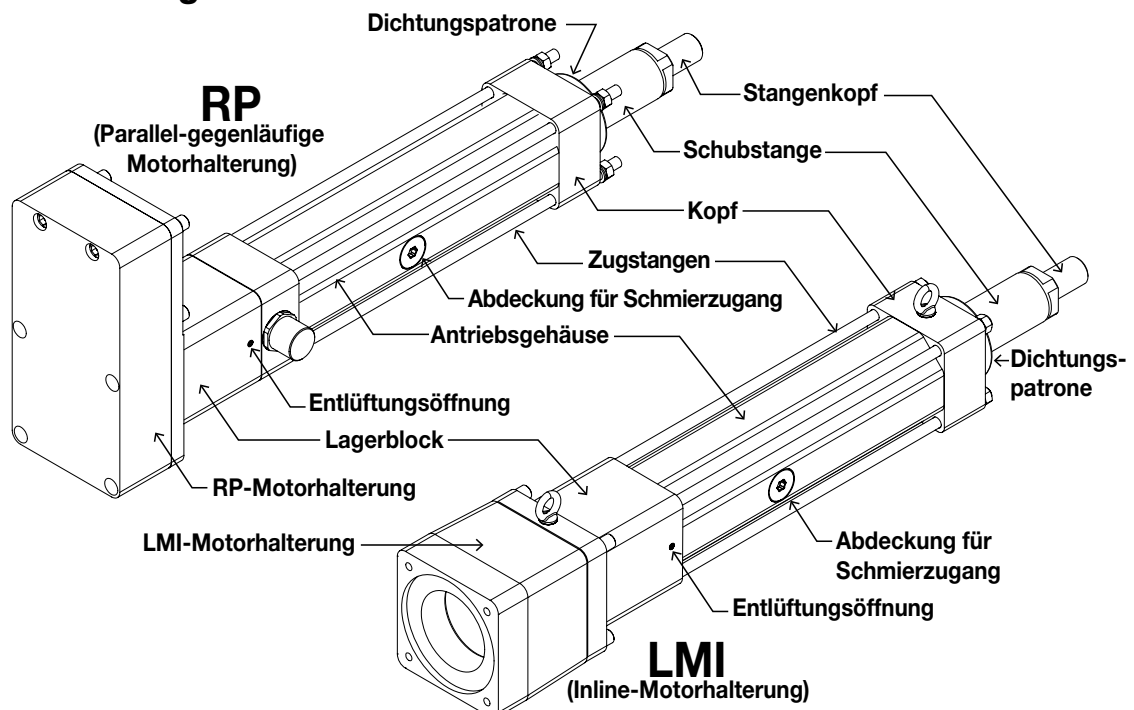
Abbildung 2-2: RSX-Stellantrieb-Hauptkomponenten
