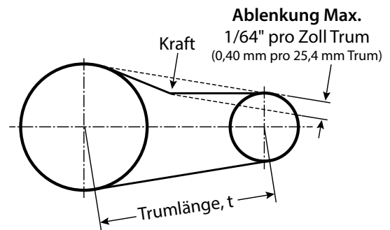
Abbildung 4-4 RSX Riemenrollendiagramm
