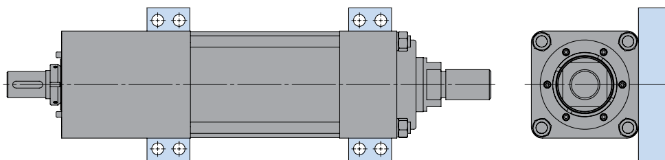
Abbildung 4-8 RSX Montageplatten-Option
