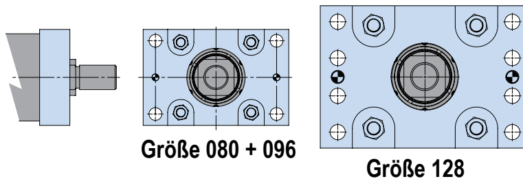
Abbildung 3-2 RSX Frontflansch-Option
